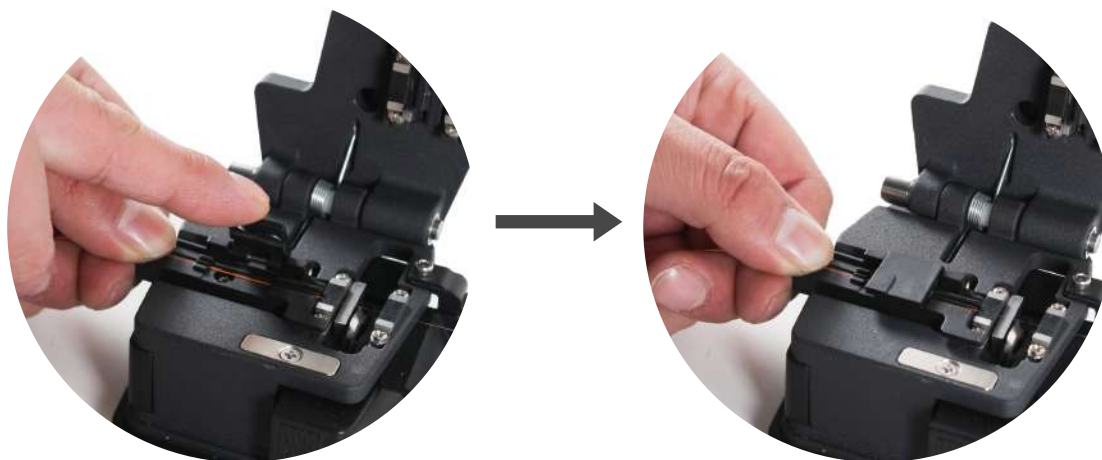
Obturador para cable de fibra abierto
